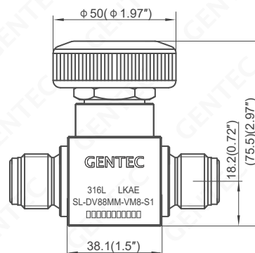
手动 (1500psi)
